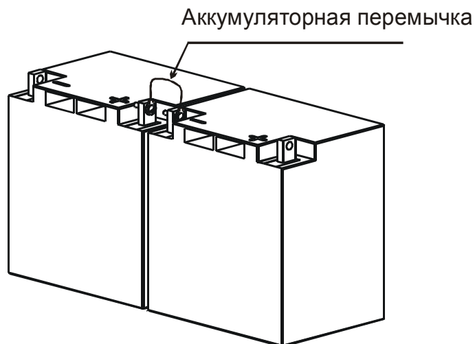
РИС.4 Схема соединения аккумуляторов
