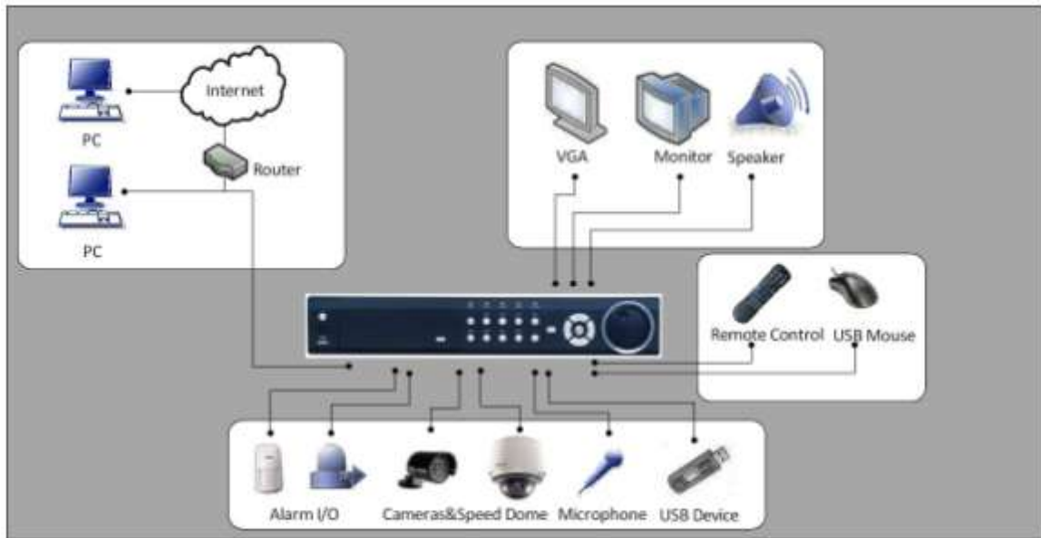
Рис. 2. Диаграмма подключений цифрового регистратора
