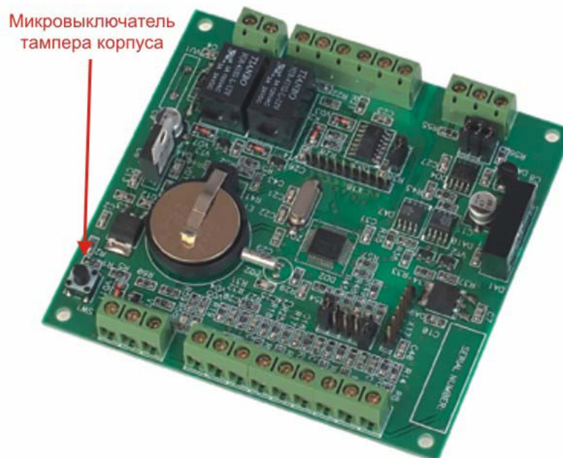
Рисунок 13. Микровыключатель тампера корпуса.
