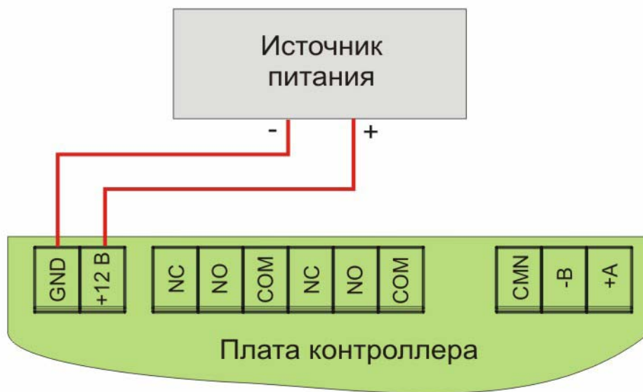
Рисунок 2. Подключение источника питания к контроллеру.
